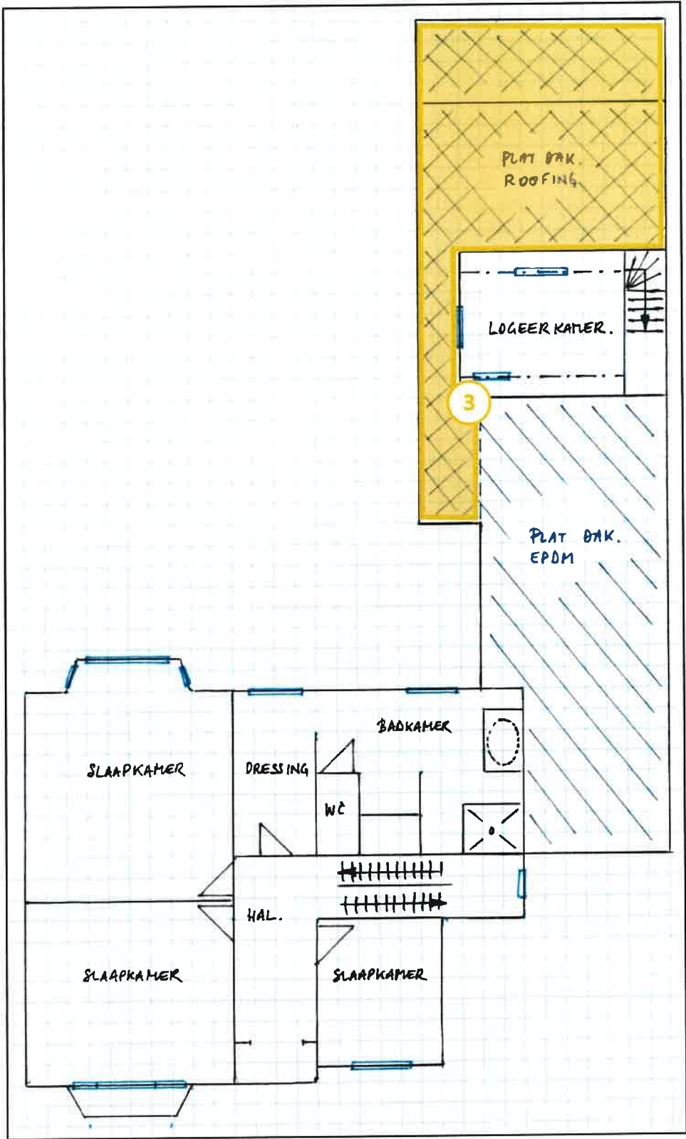
Legende van plan 1.9: Erembodegem - Brusselbaan 205 - 1e verdieping
