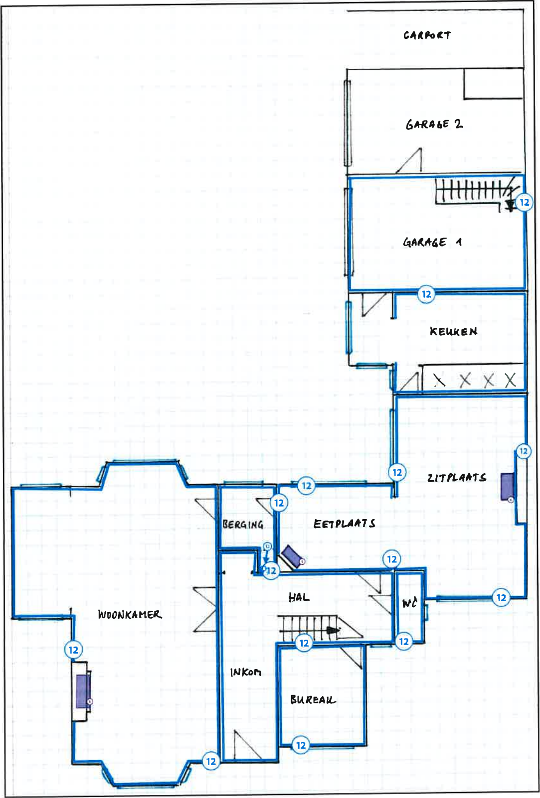
Legende van plan 1.5: Erembodegem - Brusselbaan 205 - Gelijkvloers
