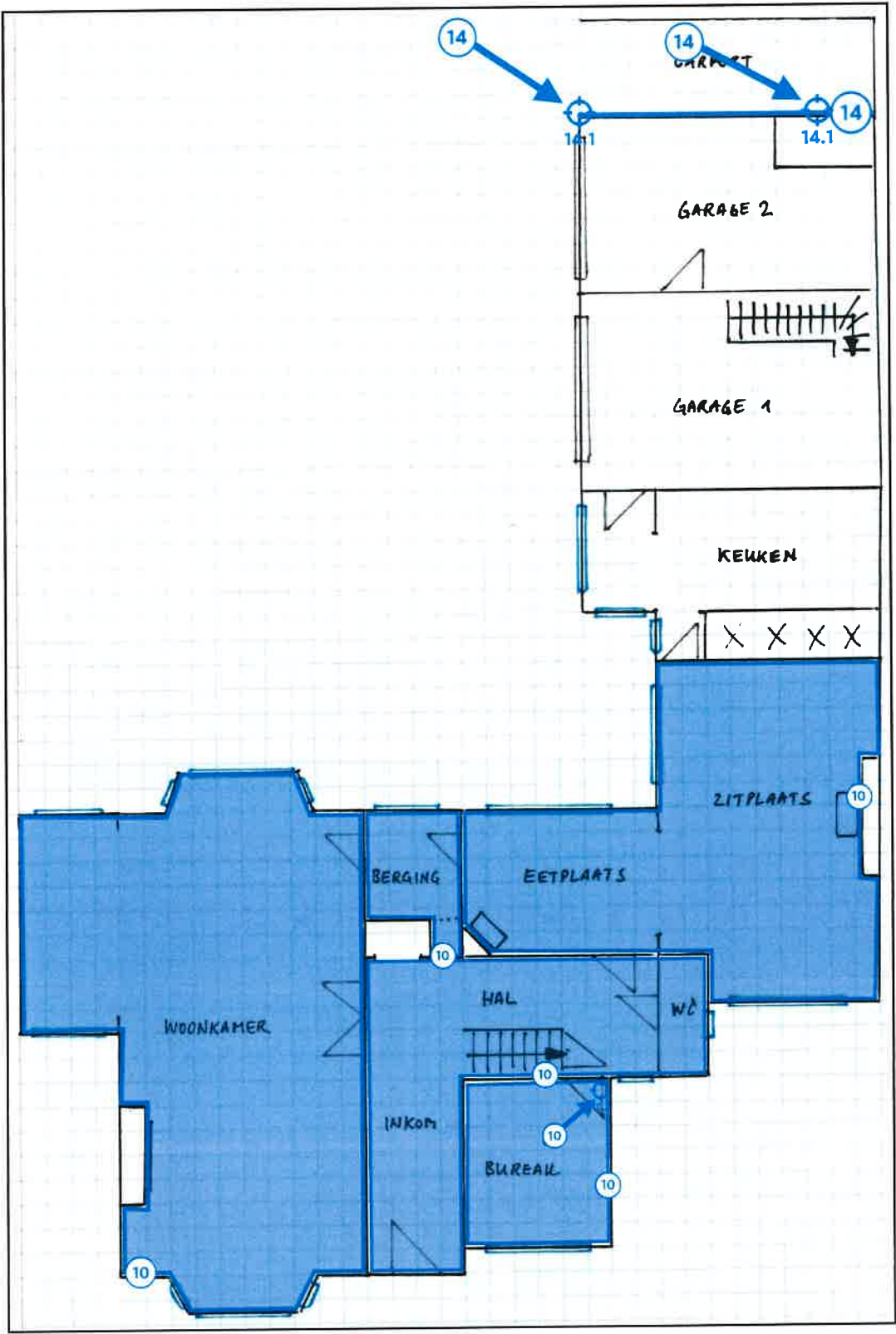
Legende van plan 1.6: Erembodegem - Brusselbaan 205 - Gelijkvloers
