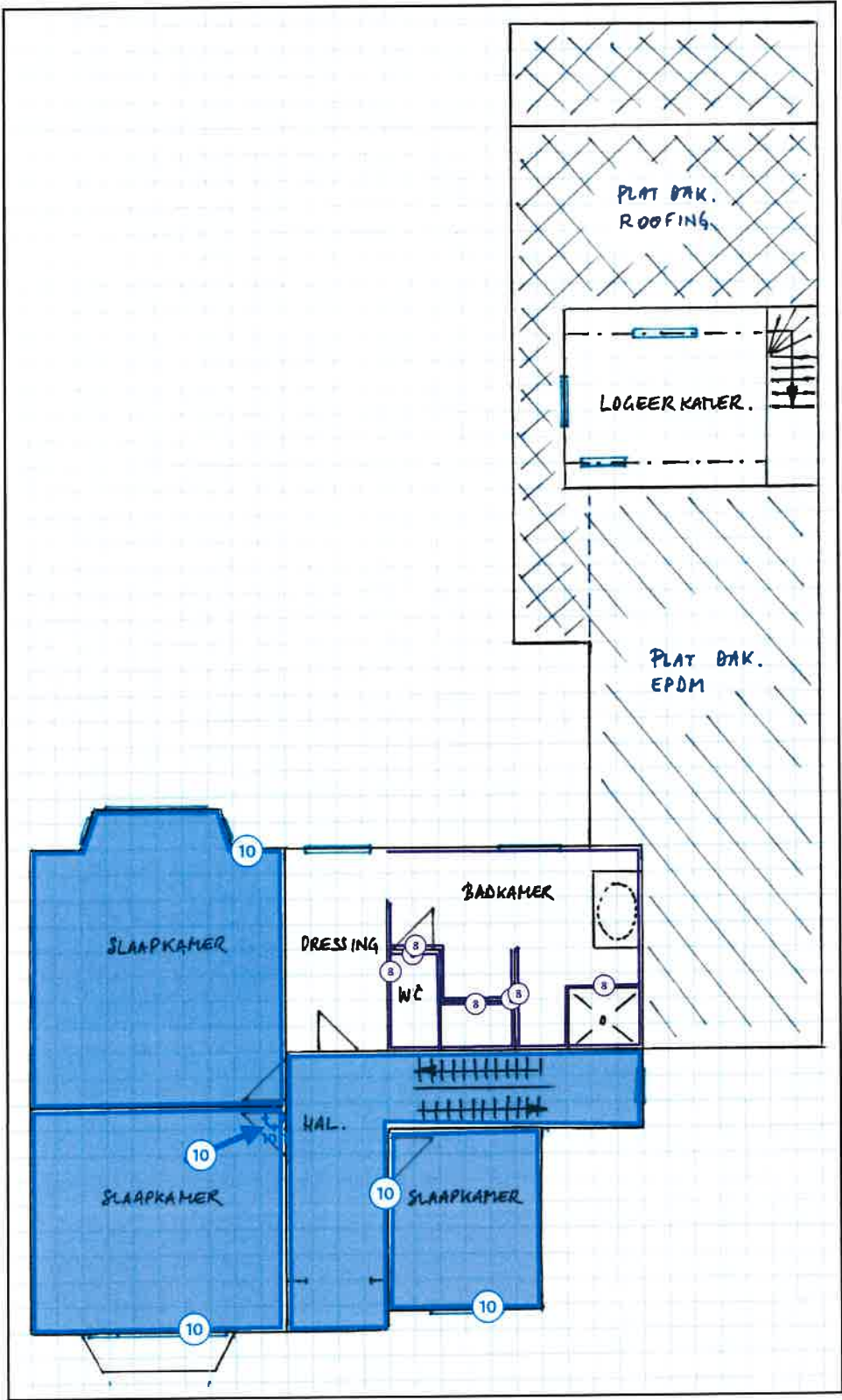
Legende van plan 1.8: Erembodegem - Brusselbaan 205 - 1e verdieping
